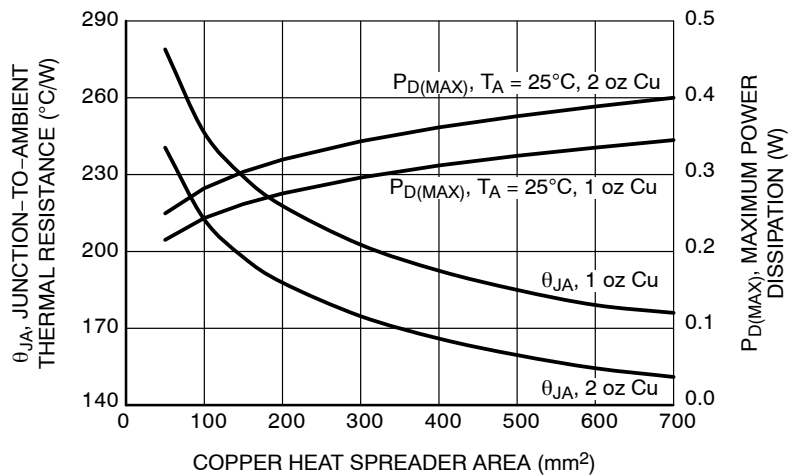
Figure 45. θ JA vs. Copper Area (uDFN4)
